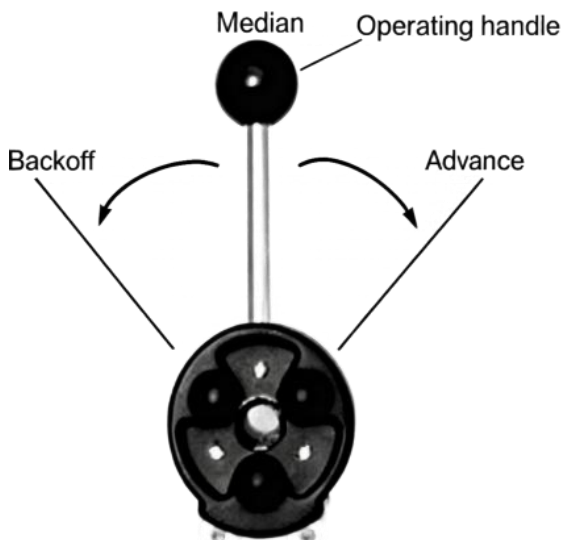
Afbeelding - Positie van de handgreep van de automatische kabelaanvoerinrichting (gezien vanaf de voorkant van de machine)
