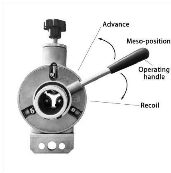
bild - Handtagsposition för automatisk kabelmatning (sett från maskinens framsida)
