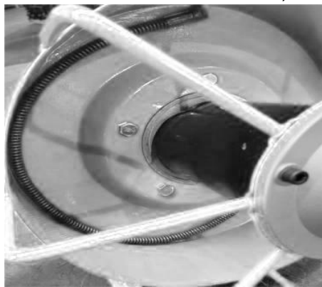
Figur 1 — Riktningen på stålvdjerns lindning inuti trumman (lindningsriktningen är svår att se på en plasttrumma, så en öppen trumma
