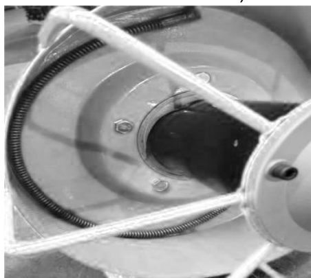
Figura 1 — Direzione dell'avvolgimento del cavo d'acciaio all'interno del tamburo (la direzione dell'avvolgimento è difficile da vedere su un tamburo di plastica, quindi per la dimostrazione viene utilizzato un tamburo aperto).
