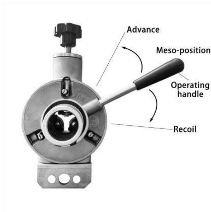
Image - Position de la poignée du dispositif d'alimentation automatique du câble (vue de face)
