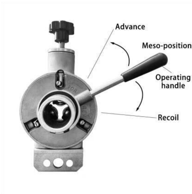
Abbildung – Position des Griffs der automatischen Kabelzuführungsvorrichtung (von der Vorderseite der Maschine aus betrachtet)
